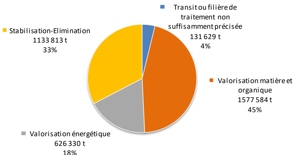
Figure 49 : Répartition par filières de traitement des DAE non dangereux non inertes d'origine régionale
